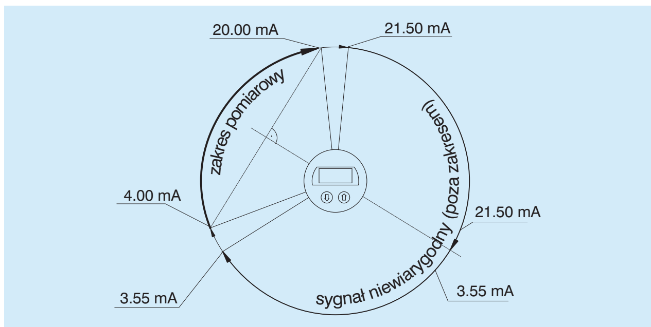
Rysunek 1. Zakres pomiarowy i sygnał niewiarygodny TRANSOLVER'a.
